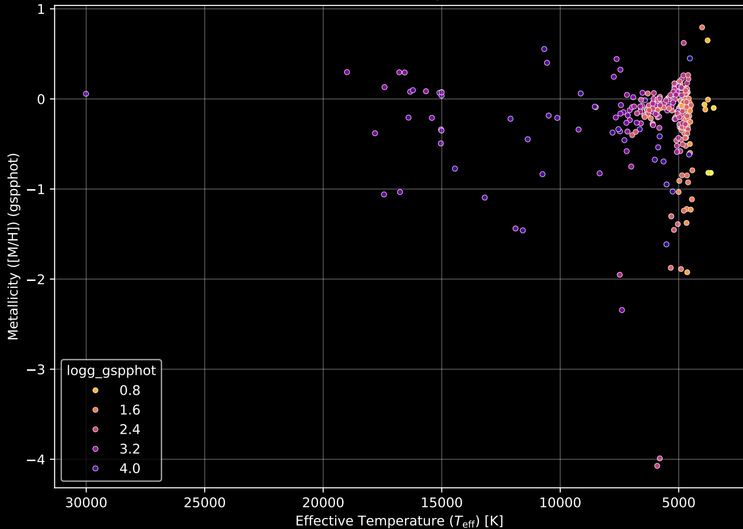
APOGEE DR17 Field: [124+00] Stellar Population Parameters (n= 282)
